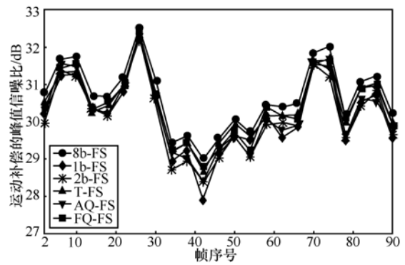
(d) Paris 序列的重构 PSNR 对比
