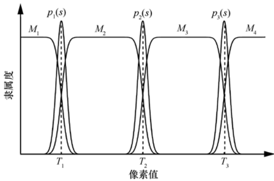
图 1 隶属度函数
